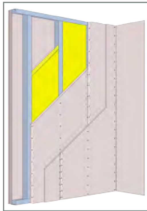
Щендерна стена с двуслойна облицовка
